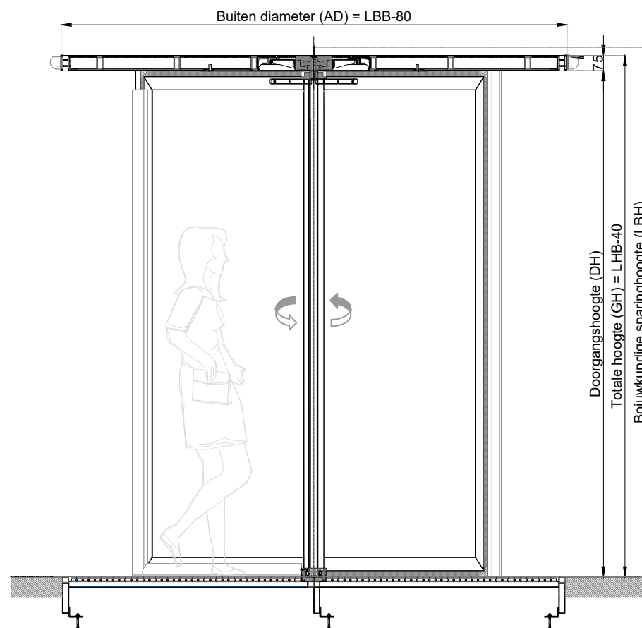
Doorsnede B-B
