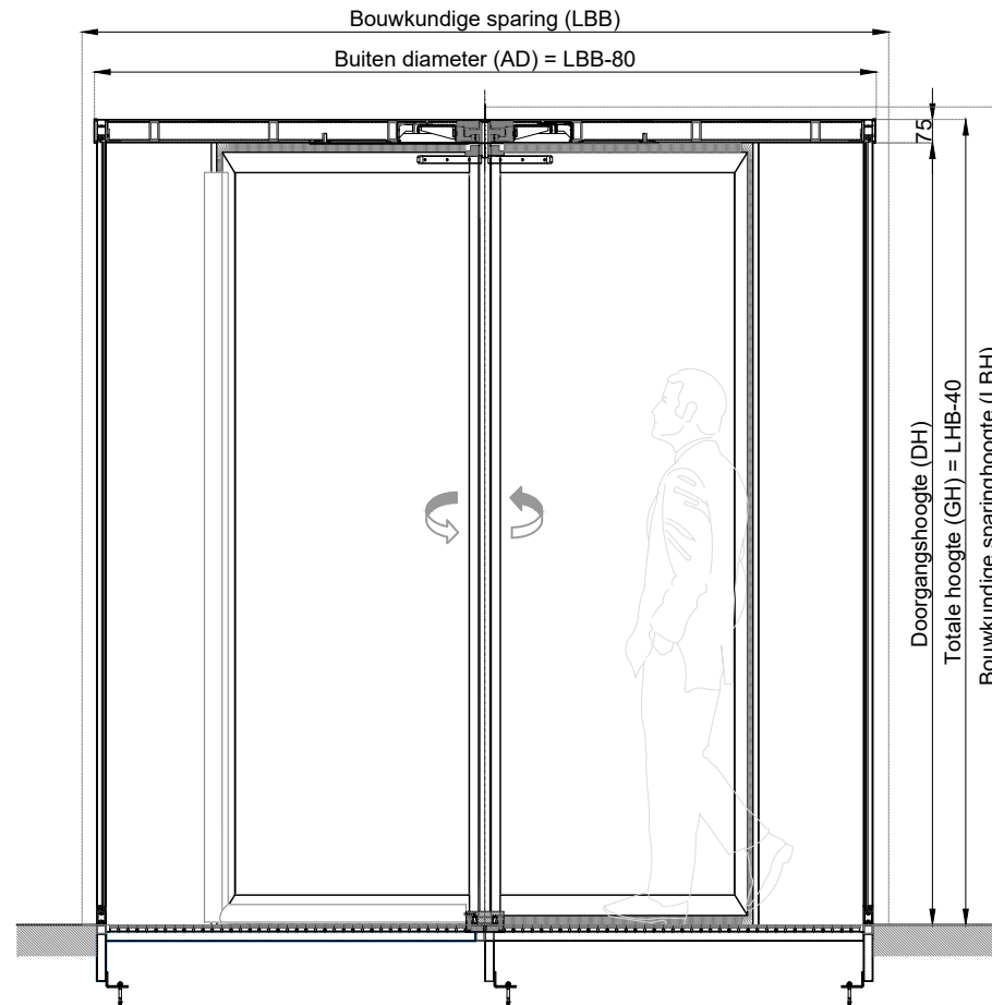
Doorsnede A-A
