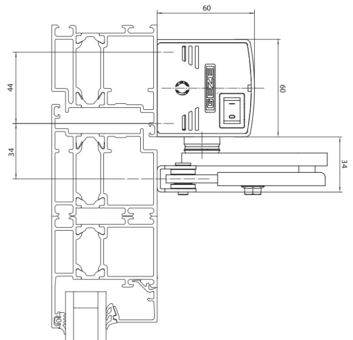
Installatie met schaararm
