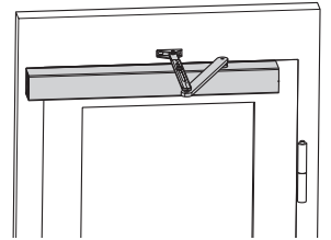
Deurblad montage met schaararm
