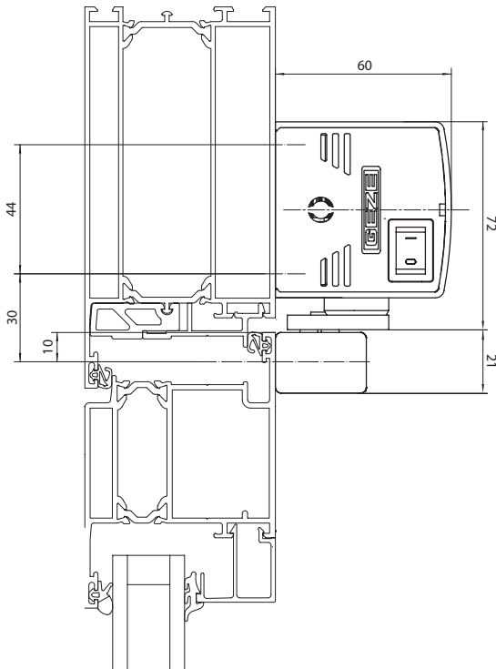
Installatie met glijrail
