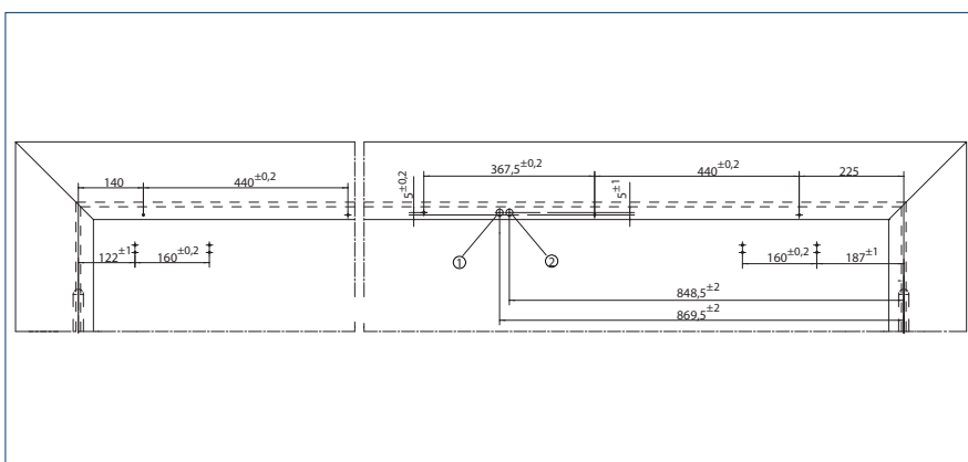
Aanslagmaten rechtermvleugel = standdeur, linkervleugel = loopdeur | 1 = ø 15 extra kabel | 2 = ø 15 230 V AC
