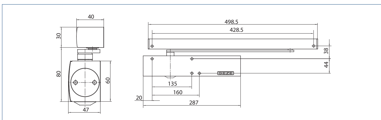
TS 5000 L-E
