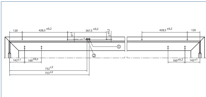
Aanslagmaten rechtermvleugel = standdeur, linkervleugel = loopdeur | 1 = ø 15 extra kabel (E-ISM / R-ISM) | 2 = ø 15 230 V AC (R-ISM)
