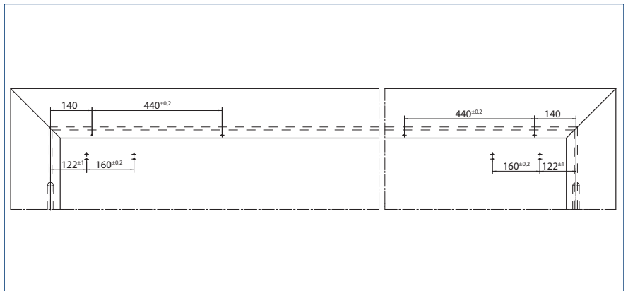
Aanslagmaten rechtere vleugel = loopdeur, linkervleugel = standdeur
