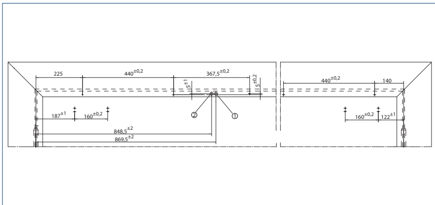
Aanslagmaten rechtermvleugel = loopdeur, linkervleugel = standdeur | 1 = ø 15 extra kabel | 2 = ø 15 230 V AC
