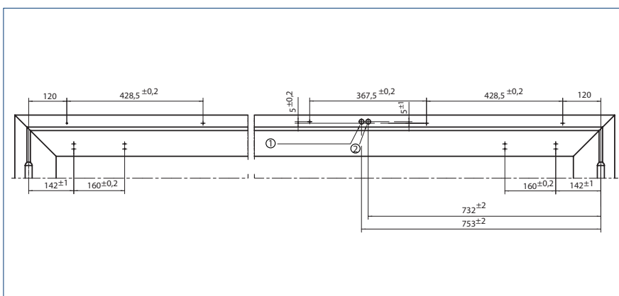
Aanslagmaten rechtermvleugel = loopdeur, linkervleugel = standdeur | 1 = ø 15 extra kabel (E-ISM / R-ISM) | 2 = ø 15 230 V AC (R-ISM)
