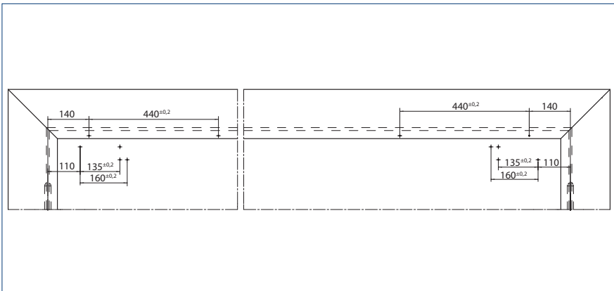
Aanslagmaten rechtereule = standeur, linkereule = loopdeur
