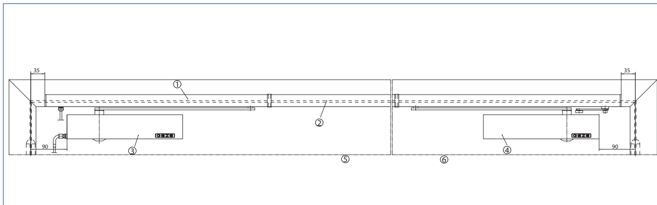
Voorbeeld voor de montage | 1 = R-ISM-glijrail BG | 2 = afkortbaar middendeel | 3 = TS 5000 L | 4 = rookmeldcentrale | 5 = loopdeur | 6 = standdeur
